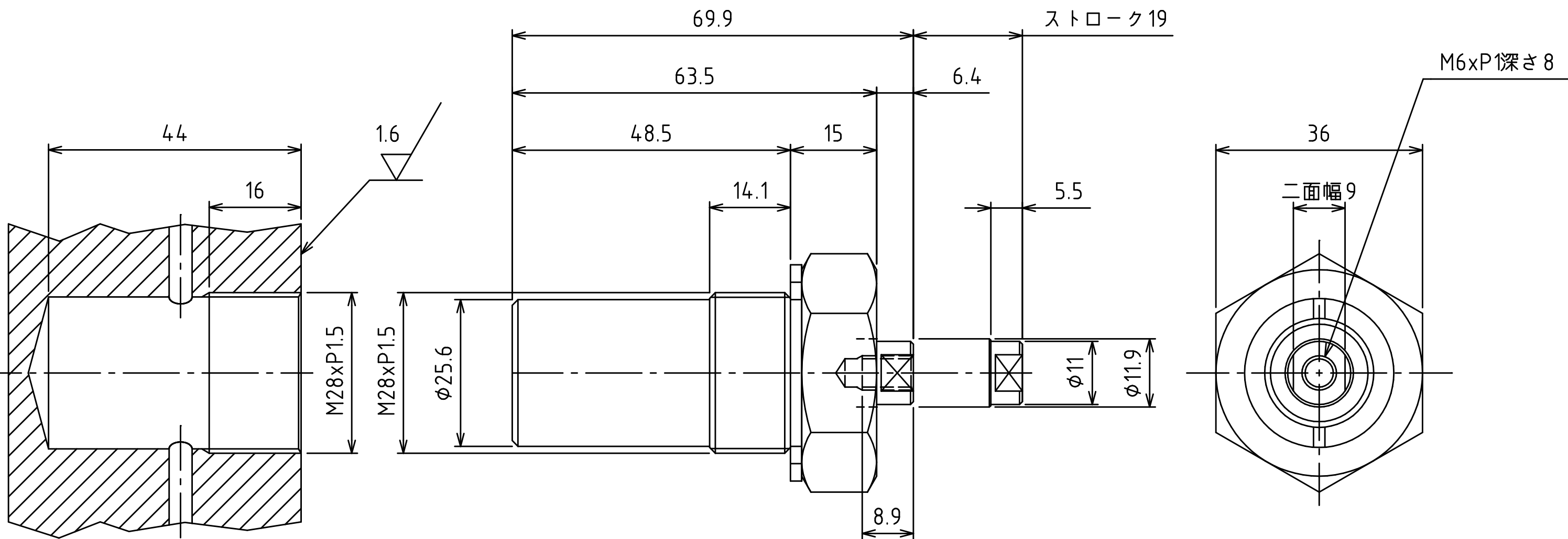
取付部加工図
