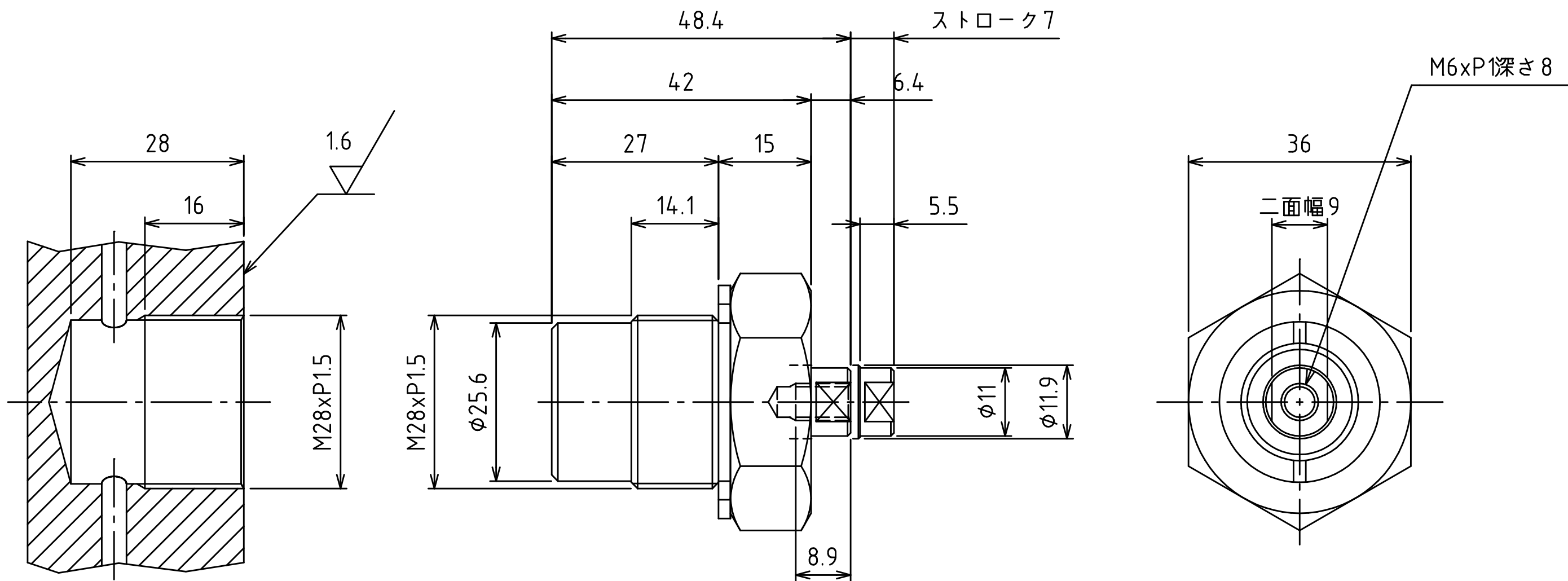
取付部加工図
