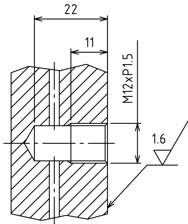
取付部加工図
