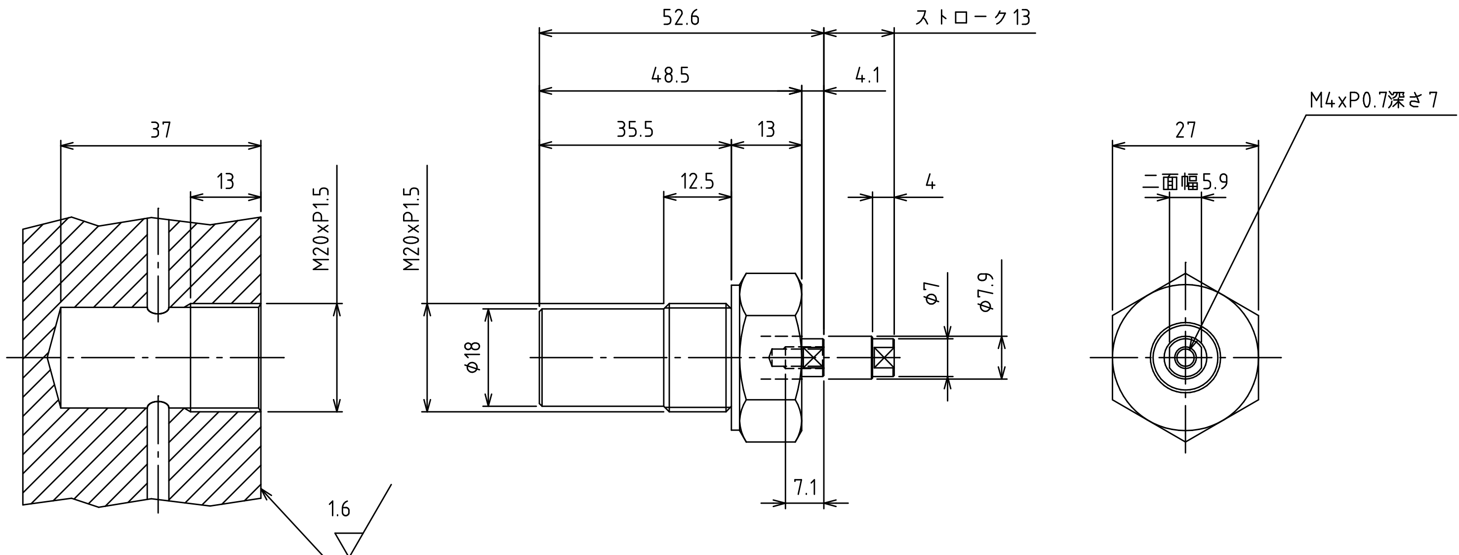
取付部加工図
