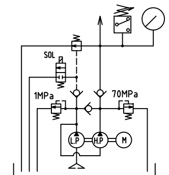
油圧回路図
