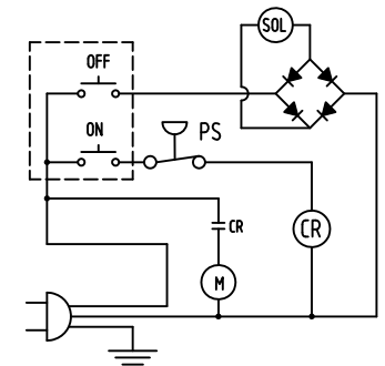
電気回路図
