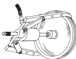
2本爪にしてプーリーの抜き作業
