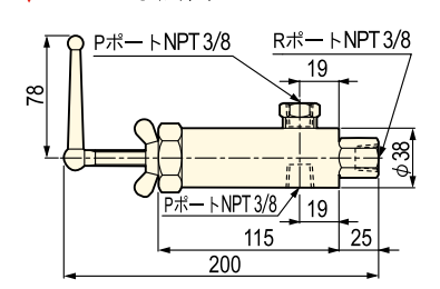
▼ V-152 寸法図
