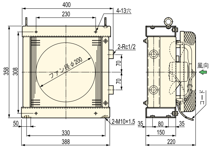
▼ W-105-02(B) 寸法図 (オイルレベルスイッチ)
