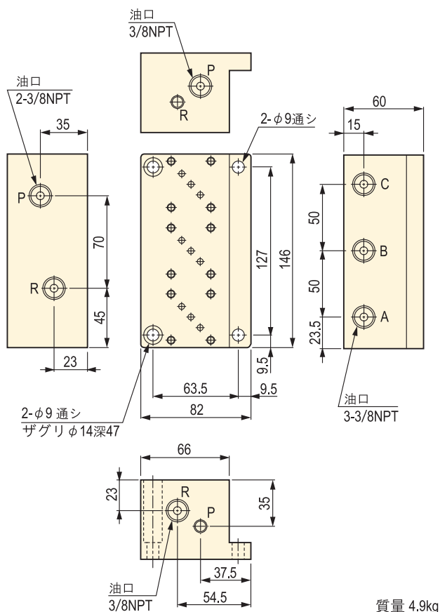
▼ WVP-3R (外部配管用)
