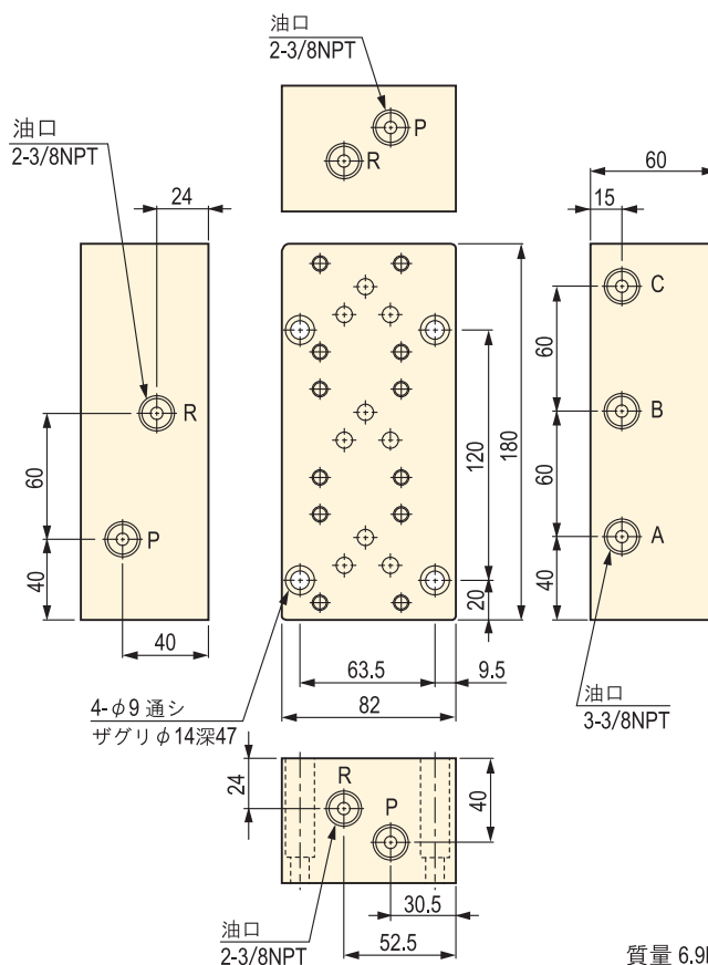
▼ WVPL-3R (外部配管用)
