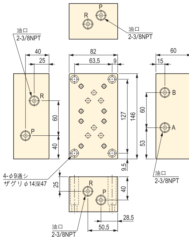
▼ WVPL-2R (外部配管用)
