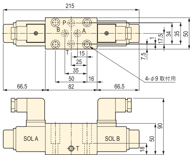
▼ VD4-O-***-10/VD4-P-***-10 寸法図
