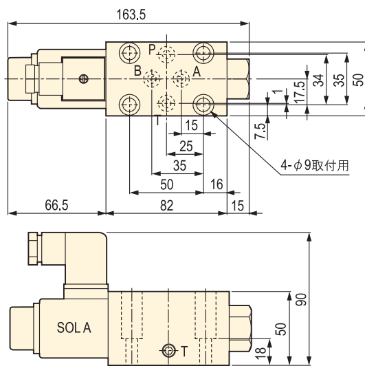
▼ VD4-N-***-10/VD4-S-***-10 寸法図
