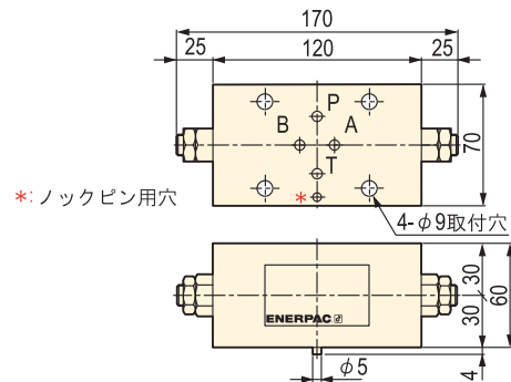
▼ VDFCD-20 (バイパス付きフローコントロールバルブ) 低油圧時のシリンダのスピード調整に使用します。
