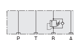
▼ 回路記号
