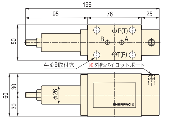
▼ VDSQ-10 (カウンタバランスバルブ) プレスでシリンダの自重落下を防止します。
