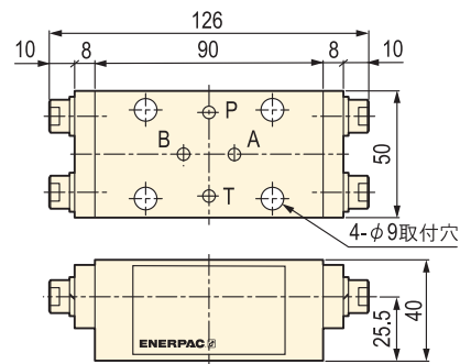
▼ 回路記号
