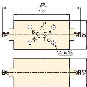
▼ VRFC40 (バイパス付フローコントロールバルブ) 低油圧時のシリンダのスピード調整に使用します。 高圧時の制御とバルブの全閉はできません。
