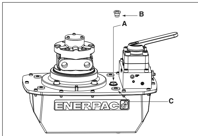
Figuur 2, ZA4 Ontluchttingsinstallatie
