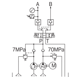
油圧回路図
