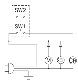
電気回路図
