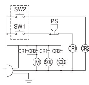
電気回路図
