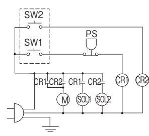
電気回路図
