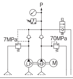
油圧回路図
