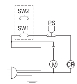
電気回路図
