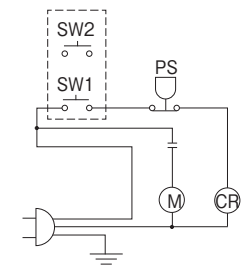
電気回路図
