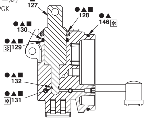
断面 A-A
