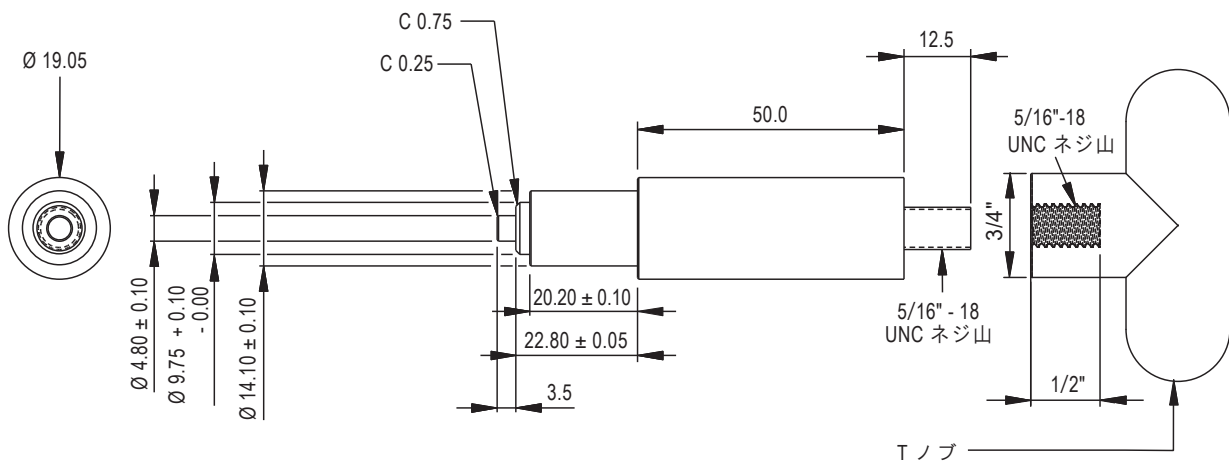
図-4 リテーニングリング取付治具 (図のように製作してください。)
