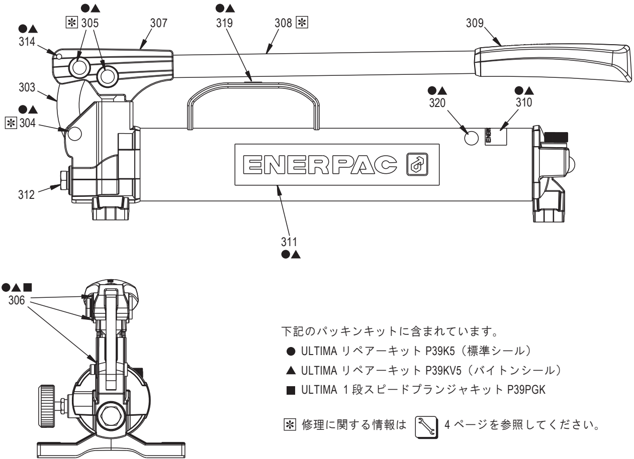
図 -1 ビーム、ハンドル、ラベル
