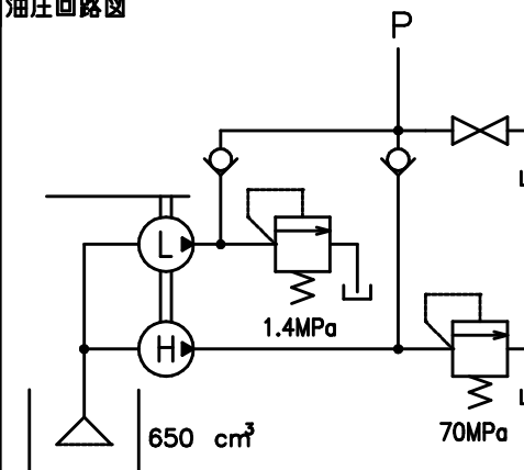
油圧回路図
