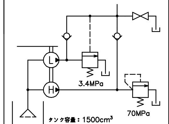
油圧回路図
