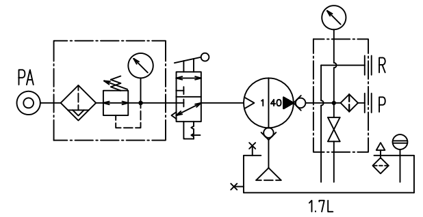
ユニット回路図
