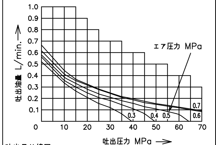
吐出量曲線図
