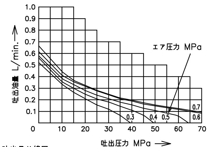
吐出量曲線図
