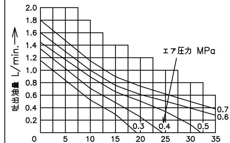
吐出量曲線図
