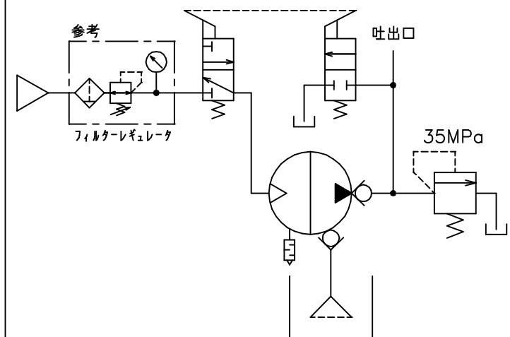
油空圧回路図
