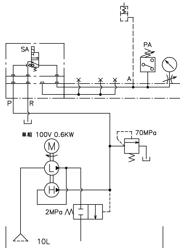
油圧回路図
