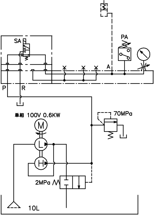
油圧回路図
