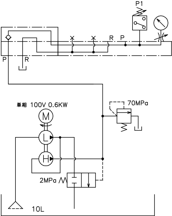
油圧回路図
