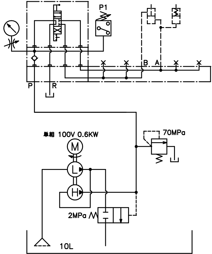
油圧回路図
