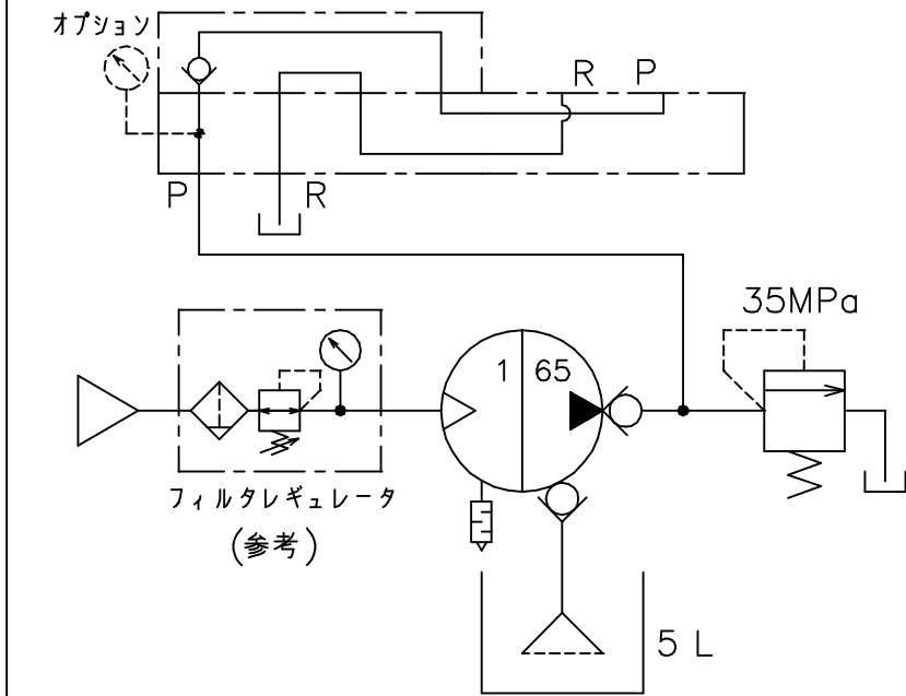
油空圧回路図
