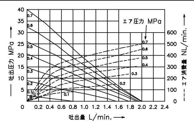
吐出量曲線図
