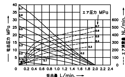
吐出量曲線図
