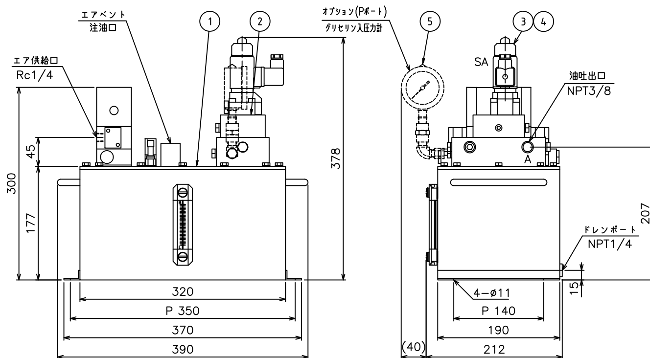
電磁弁形状 (ZAJ06505-S1C)
