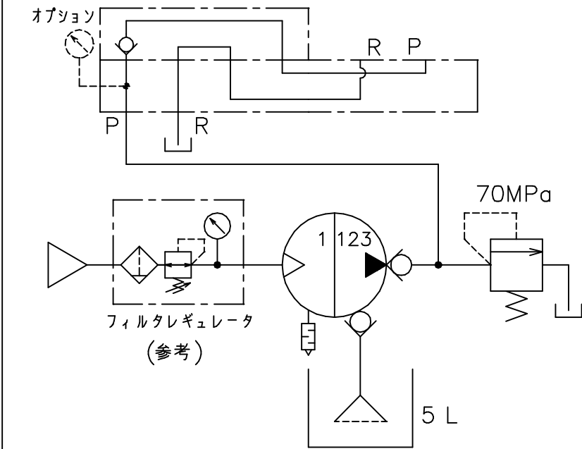
油空圧回路図
