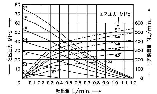
吐出量曲線図
