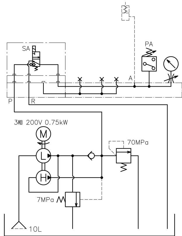
油圧回路図
