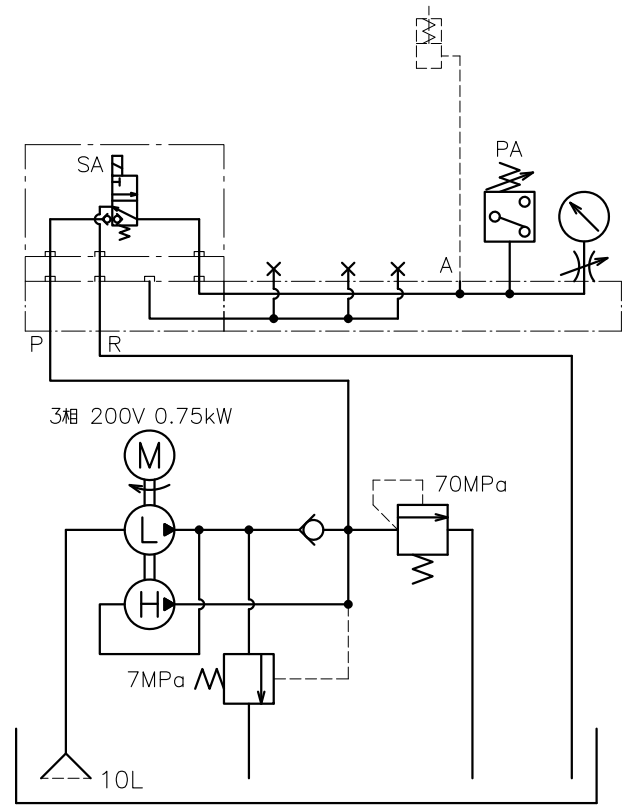
油圧回路図
