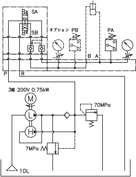
油圧回路図
