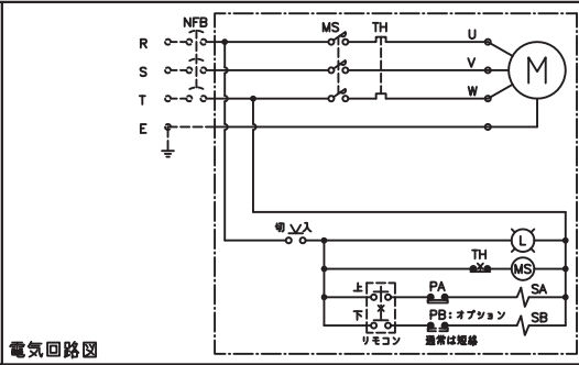
電気回路図
