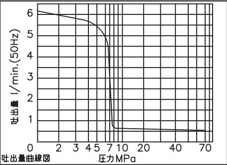
吐出量曲線図
