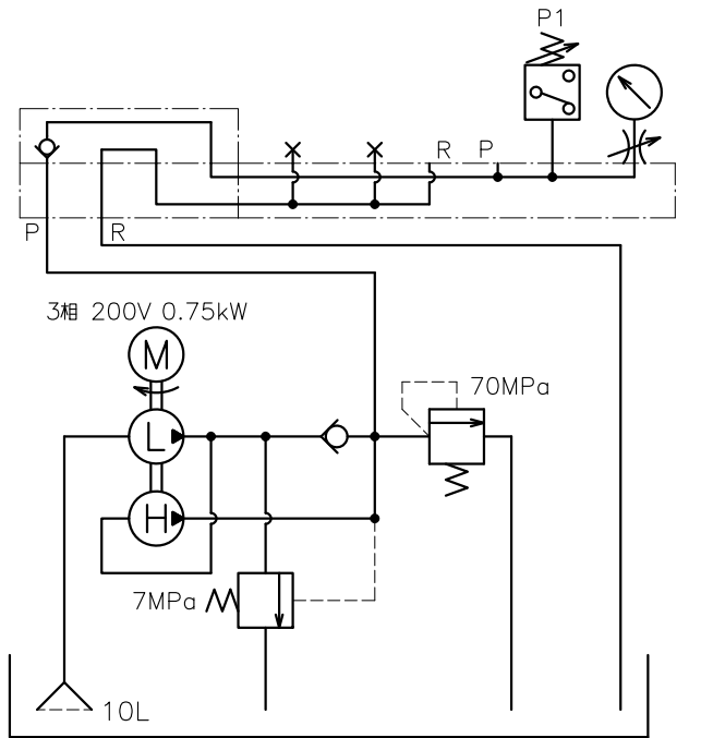
油圧回路図
