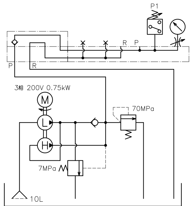
油圧回路図
