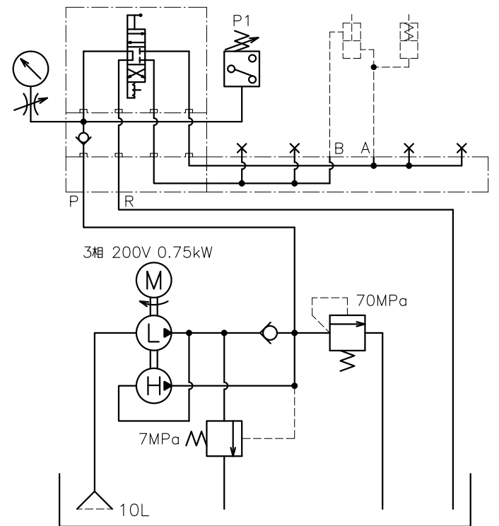
油圧回路図
