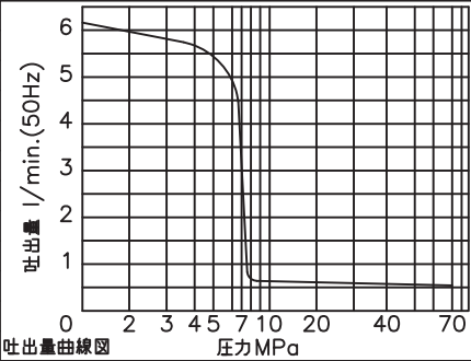
吐出量曲線図
