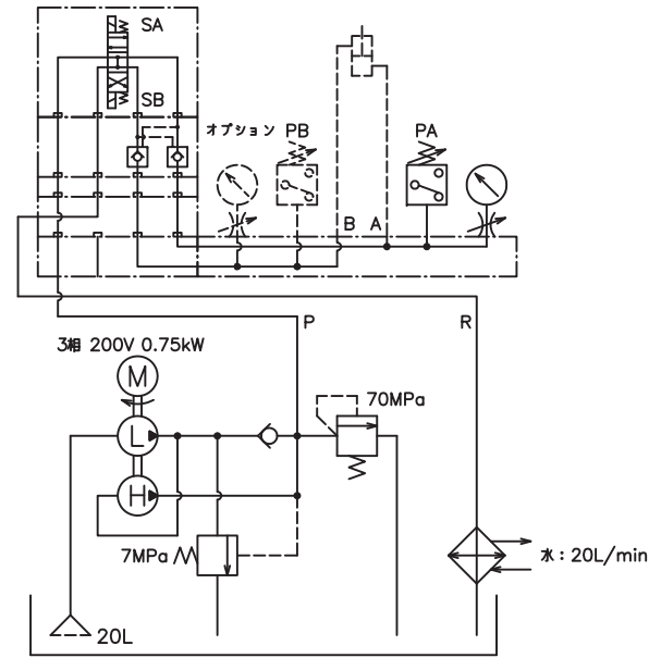
油压回路图
