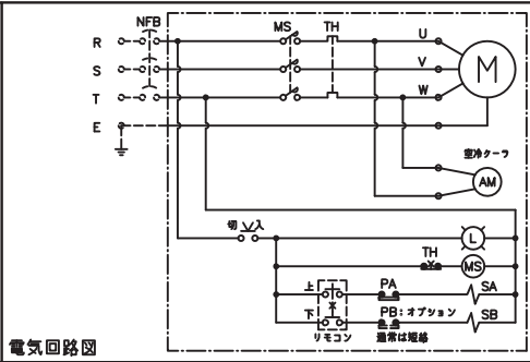
電気回路図
