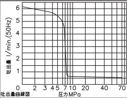
吐出量曲線図
