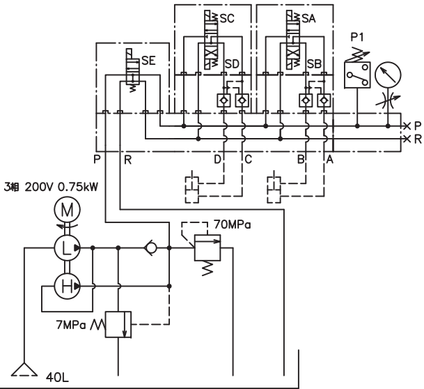
油圧回路図
