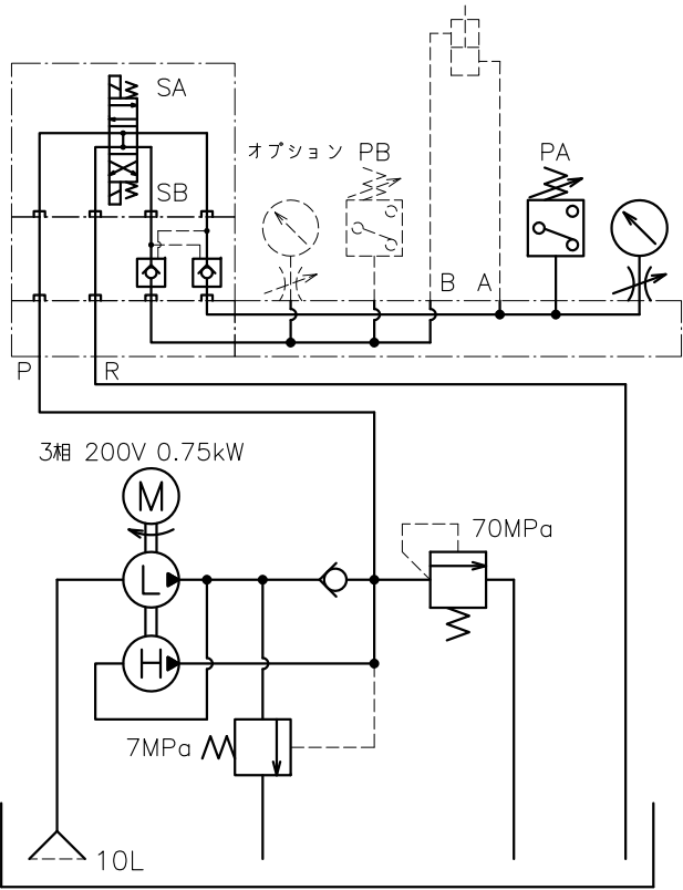
油圧回路図
