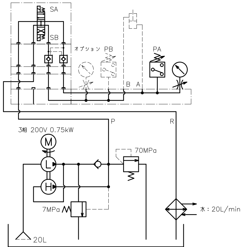
油圧回路図
