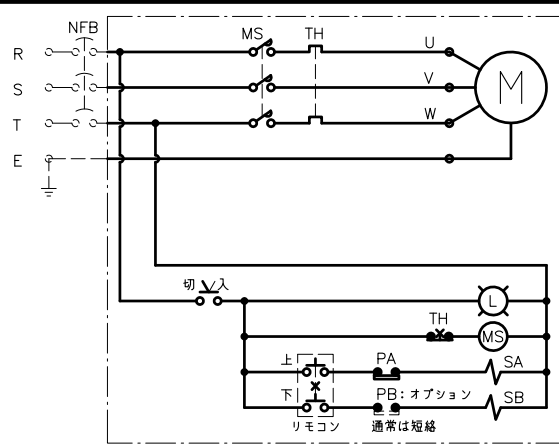
電気回路図
