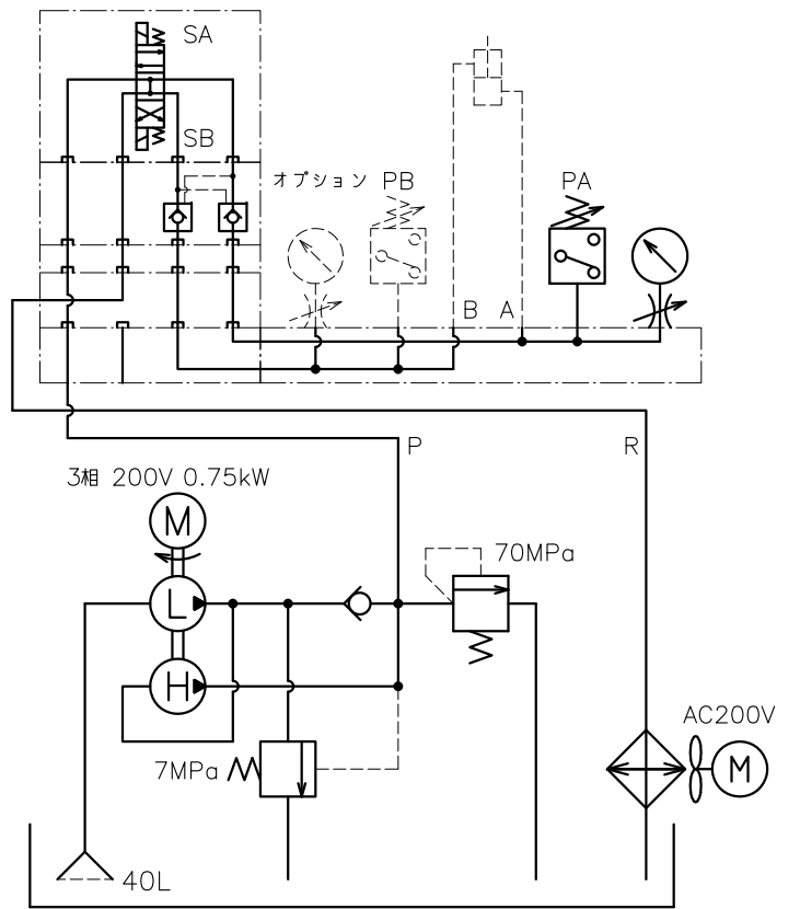
油圧回路図
