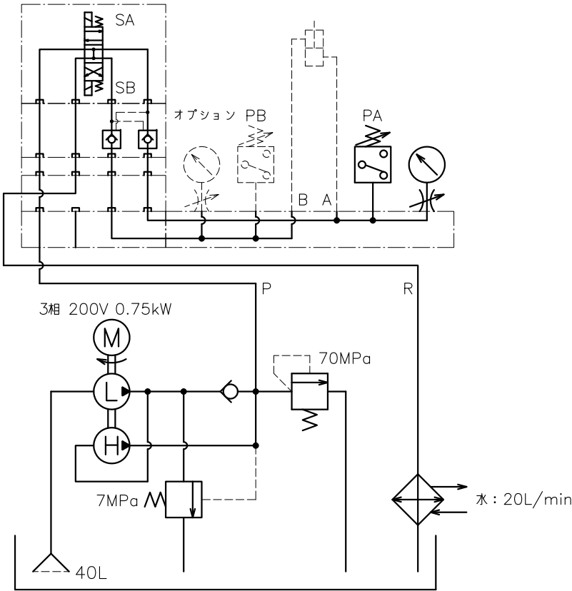
油圧回路図
