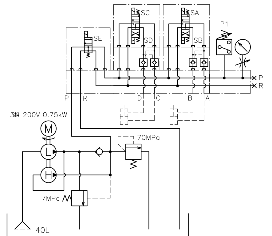
油压回路图
