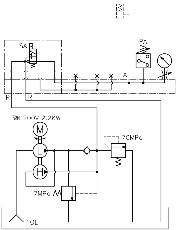
油圧回路図
