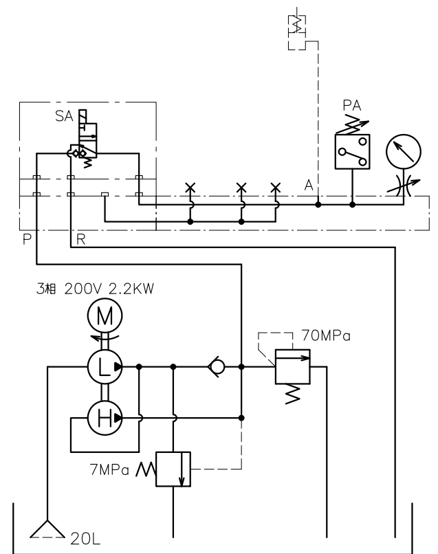
油圧回路図
